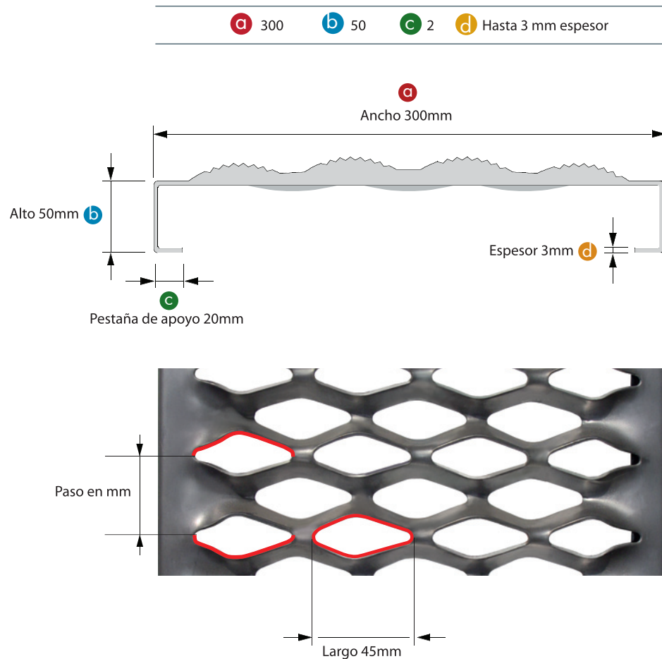
Dimensiones piso Perfilado P30 standart
